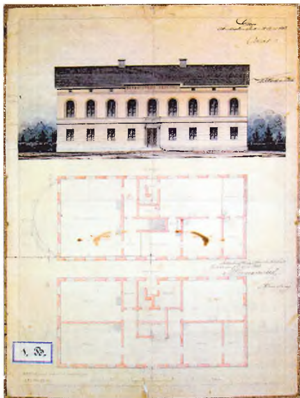
Den ursprungliga ritningen till läroverket från 1854. Mariestads stadsbyggnadskontor.
