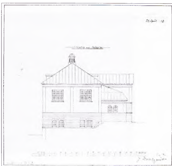
Ovan till vänster planritning över skolområdet före gymnastikbyggnadens uppförande på 1910-talet. Till höger originalritningen över gymnastikhusets södra fasad. Mariestads stadsbyggnadskontor.
