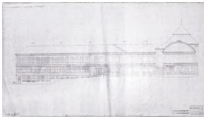
Fasadritningarna på tillbyggnaden från 1930-talet ses ovan. Överst ses fasadritningar över fasaderna mot väster överst och därunder fasaden mot öster från 1930-talet. Nedan ombyggnadsritningen över byggnad 3, Cantus Durus. Mariestads stadsbyggnadskontor.
